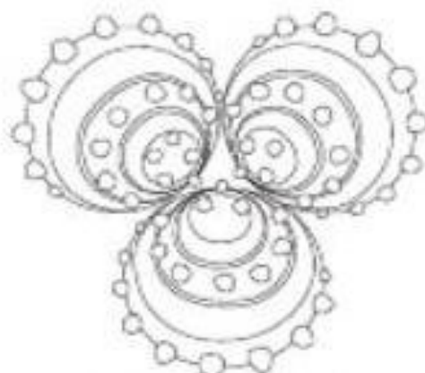
Vista de los tres conos rodantes (herramienta colocada sobre el extremo del macho)
